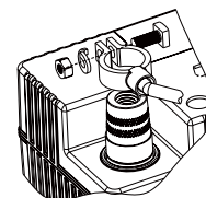
SAEタイプ自動車用端子アダプター取付け例 (品番#SHO-SAETERM)
